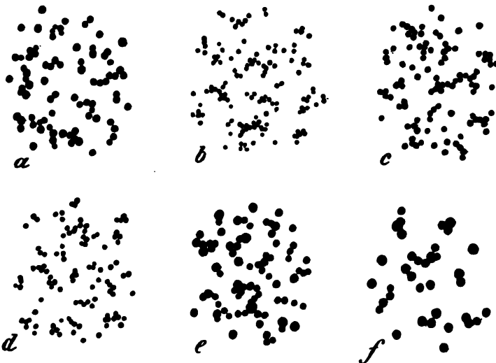
Fig. 3. Granula, aus schwach saurer, 10-proc. Albumoselösung gefällt mit a 1-proc. Platinchlorid, b 0,5 Chromsäure, c FLEMMING'scher Lösung, d 2,5 Kaliumbichromat, e MÜLLER'scher Lösung. Zum Vergleich in f , eine 3-proc., schwach saure Albumose mit 1 Proc. Osmiumsäure, die viel grössere Granula fällt. Man vergleiche auch die Tabelle und Fig. 1 und 4. (Vergr. 600.)
